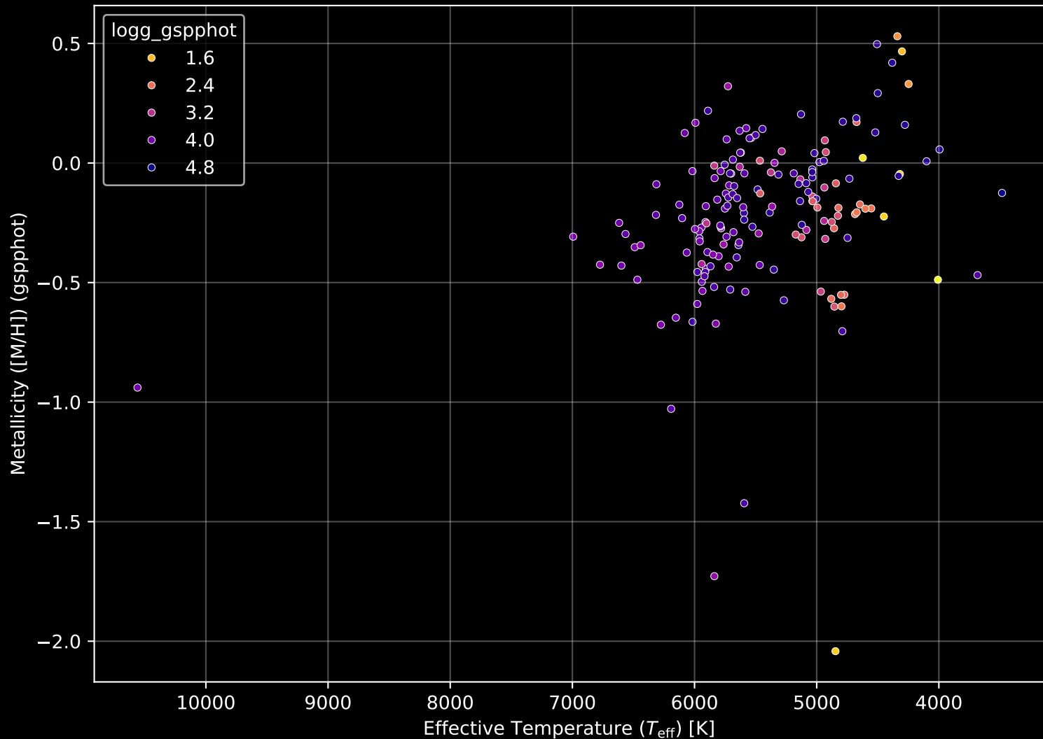
APOGEE DR17 Field: [278-39-O_TESS] Stellar Population Parameters (n= 170)
